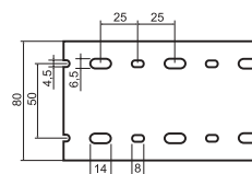
Děrování DIN ve dvou řadách od šíře 80 mm.
